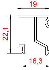
PROFİL NO : 1454 AĞIRLIK : 0.255 Kg/m
