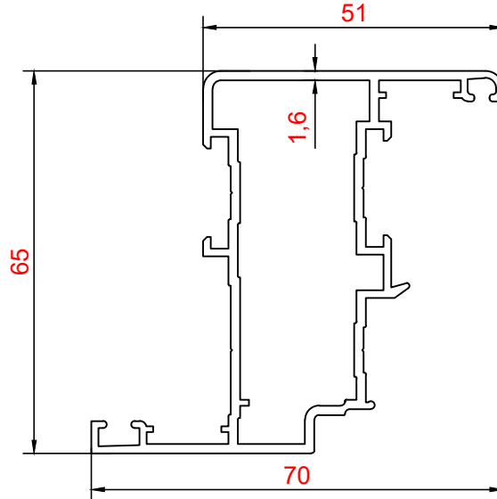
PROFİL NO : 2861 AĞIRLIK : 1.134 Kg/m
