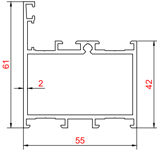
PROFİL NO : 191 AĞIRLIK : 1.214 Kg/m
