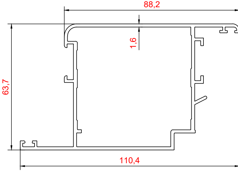
PROFİL NO : 1862 AĞIRLIK : 1.511 Kg/m
