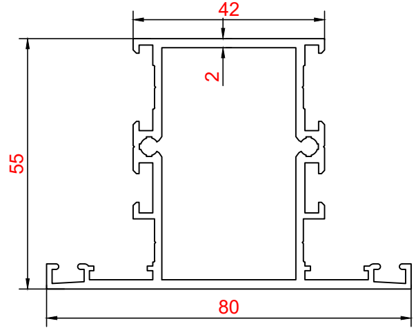
PROFİL NO : 180 AĞIRLIK : 1.377 Kg/m
