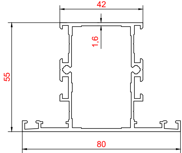
PROFİL NO : 1859 AĞIRLIK : 1.260 Kg/m
