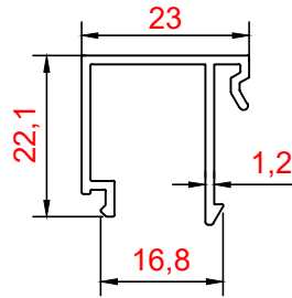
PROFİL NO : 186 AĞIRLIK : 0.256 Kg/m
