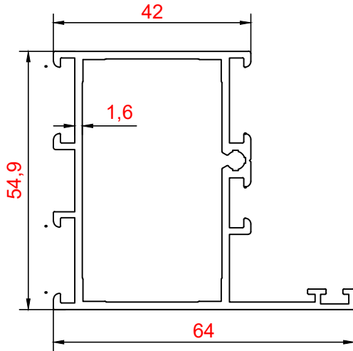
PROFİL NO : 1858 AĞIRLIK : 1.095 Kg/m
