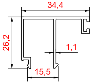
PROFİL NO : 1860 AĞIRLIK : 0.310 Kg/m
