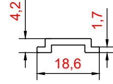
PROFİL NO : 303 AĞIRLIK : 0.117 Kg/m
