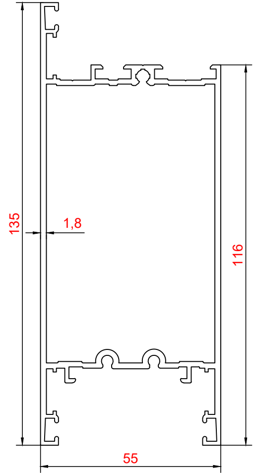
PROFİL NO : 181 AĞIRLIK : 1.977 Kg/m
