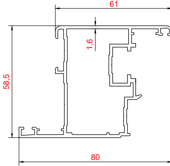
PROFİL NO : 2860 AĞIRLIK : 1.279 Kg/m
