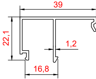
PROFİL NO : 187 AĞIRLIK : 0.308 Kg/m
