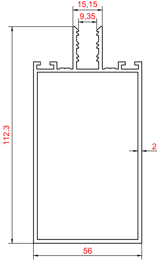
GRİYAJ PROFİLİ PROFİL NO : 2678 AĞIRLIK : 1,859 Kg/m
