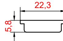
PROFİL NO : 2680 AĞIRLIK : 0,306 Kg/m
