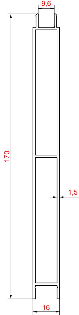
LAMBRI PROFİLİ PROFİL NO : 2486 AĞIRLIK : 1,528 Kg/m
