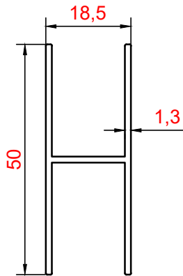
H PROFİLİ PROFİL NO : 2679 AĞIRLIK : 0,408 Kg/m
