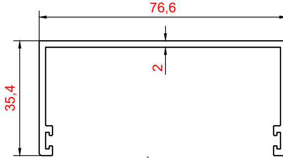
PROFİL NO : 2484 AĞIRLIK : 0,835 Kg/m
