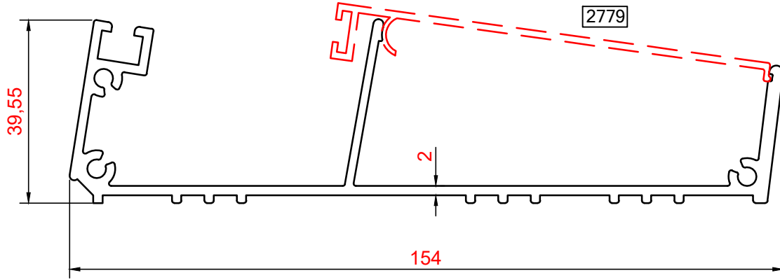
DUVAR SABİTLEME PROFİLİ PROFİL NO : 2707 AĞIRLIK : 1,771 Kg/m
