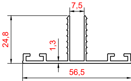
GRİYAJ KAPAK PROFİLİ PROFİL NO : 2481 AĞIRLIK : 0,425 Kg/m
