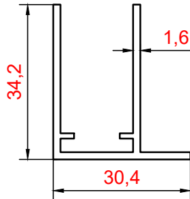
F PROFİLİ PROFİL NO : 2479 AĞIRLIK : 0,440 Kg/m
