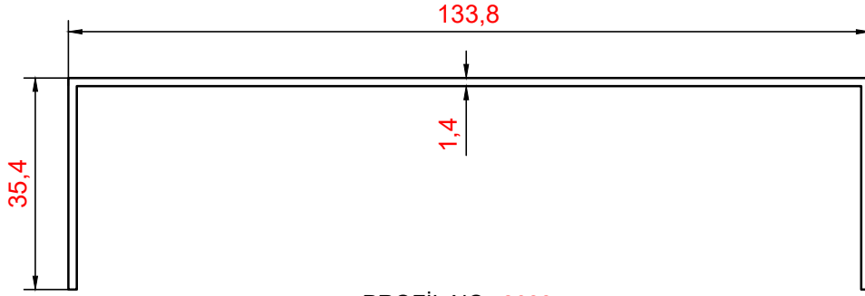
PROFİL NO : 2688 AĞIRLIK : 0,766 Kg/m
