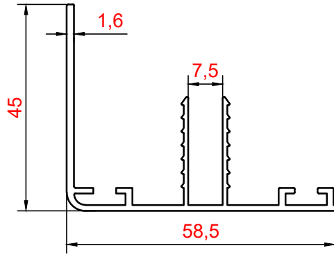
GRİYAJ KENAR KAPAK PROFİLİ PROFİL NO : 2480 AĞIRLIK : 0,606 Kg/m
