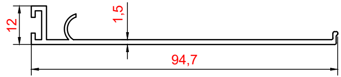
OLUK KAPAK PROFİLİ PROFİL NO : 2478 AĞIRLIK : 0,485 Kg/m
