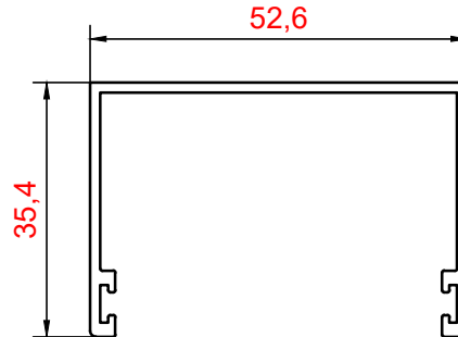
PROFİL NO : 2739 AĞIRLIK : 0,513 Kg/m
