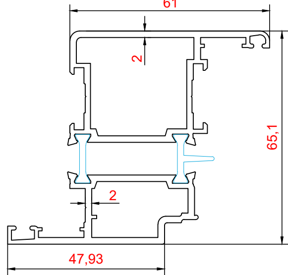
KANAT PROFİLİ
