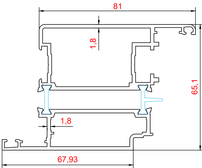
KANAT PROFİLİ
