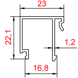
PROFİL NO : 186 AĞIRLIK : 0.255 Kg/m
