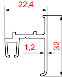
PROFİL NO : 2878 AĞIRLIK : 0.298 Kg/m
