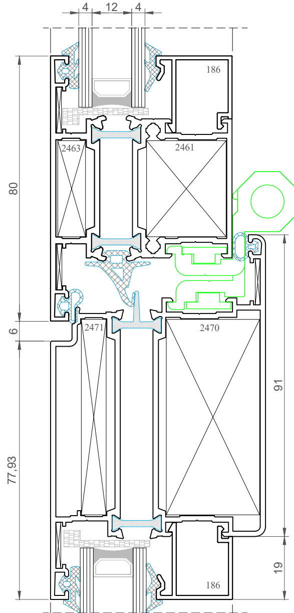
DETAY DETAY 2
