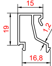
PROFİL NO : 2879 AĞIRLIK : 0.244 Kg/m
