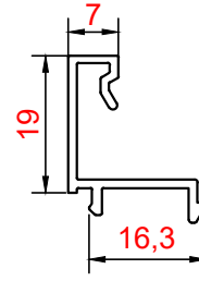
PROFİL NO : 2880 AĞIRLIK : 0.190 Kg/m
