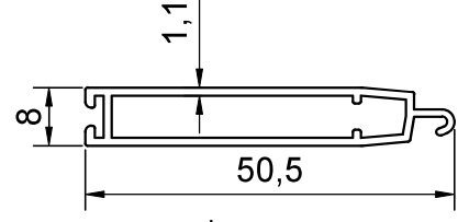
PROFİL NO : 1506 AĞIRLIK : 0.339 Kg/m
