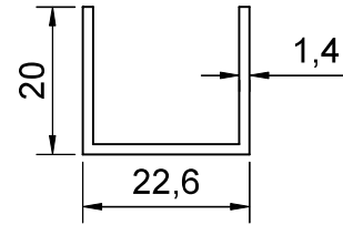
PROFİL NO : 2284 AĞIRLIK : 0.228 Kg/m
