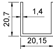
PROFİL NO : 2285 AĞIRLIK : 0.222 Kg/m
