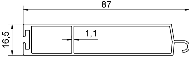
PROFİL NO : 298 AĞIRLIK : 0.694 Kg/m
