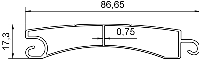
PROFİL NO : 1622 AĞIRLIK : 0.528 Kg/m
