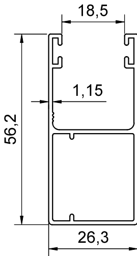
PROFİL NO : 1464 AĞIRLIK : 0.575 Kg/m
