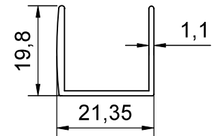
PROFİL NO : 1432 AĞIRLIK : 0.195 Kg/m
