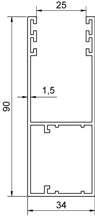
PROFİL NO : 290 AĞIRLIK : 1.182 Kg/m
