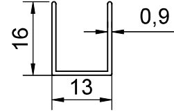
PROFİL NO : 1328 AĞIRLIK : 0.106 Kg/m
