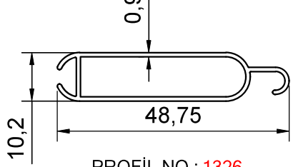
PROFİL NO : 1326 AĞIRLIK : 0.268 Kg/m
