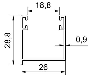
PROFİL NO : 1327 AĞIRLIK : 0.241 Kg/m
