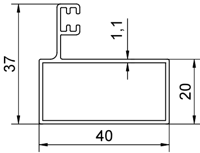
PROFİL NO : 323 AĞIRLIK : 0.453 Kg/m
