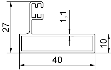
PROFİL NO : 349 AĞIRLIK : 0.393 Kg/m
