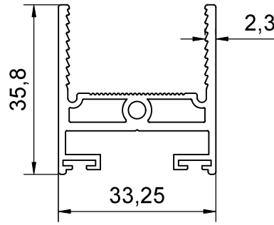
PROFİL NO : 1532 AĞIRLIK : 0.726 Kg/m
